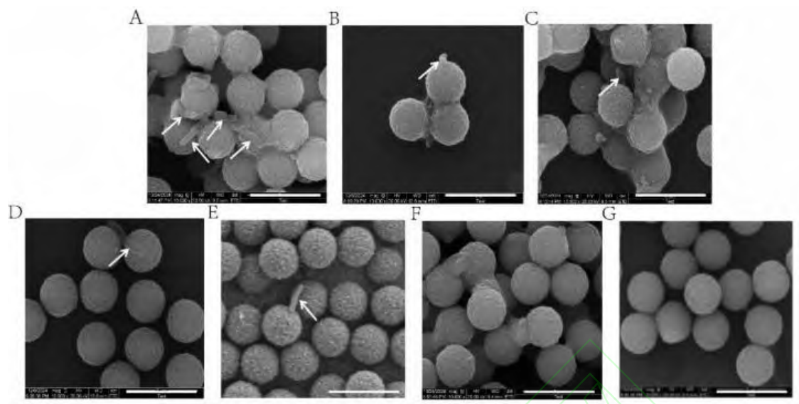
图 2 免疫磁珠捕获的游离 H. pylori 的 SEM 照片 \times 10\,000
