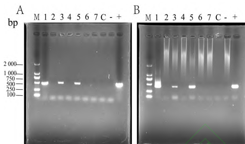
图3 免疫磁珠复合物中存在 H. pylori 特异性基因 16S rDNA、 ureA
