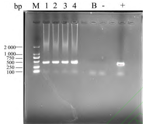
图 1 PCR 检测念珠菌内 H. pylori ureA 基因
