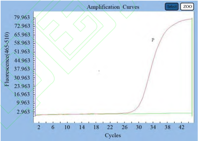
图 1 4 株菌株的 qPCR 扩增曲线
