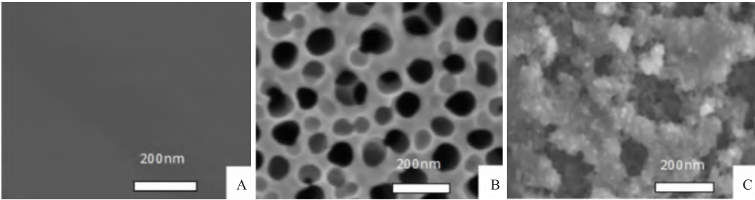
图1 纯钛片和钛纳米管形貌 ×30 000
