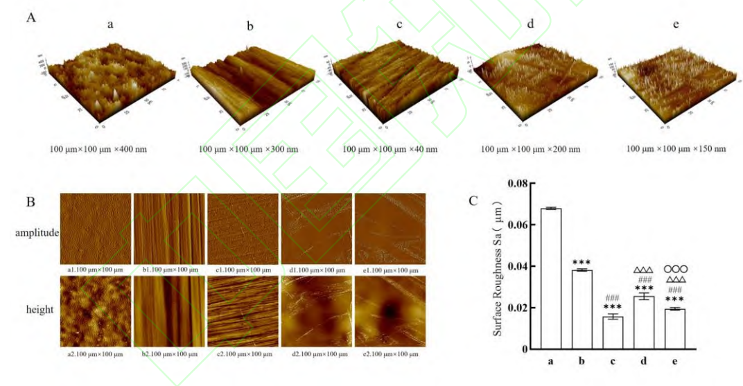
图 1 表面粗糙度的测定及结果
