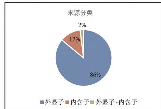
图 4 根据基因组起源对显著失调的 circRNAs 进行分类
