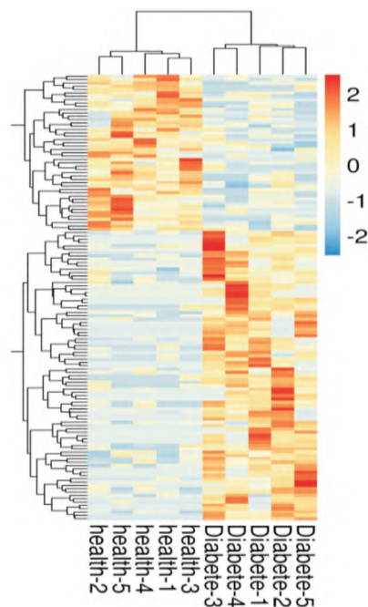
图 3 NC 和 T2DM 外周血微阵列分析热图
