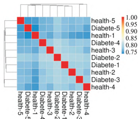
图2 样本聚类图
