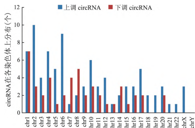
图 5 染色体中环状 RNA 分布
