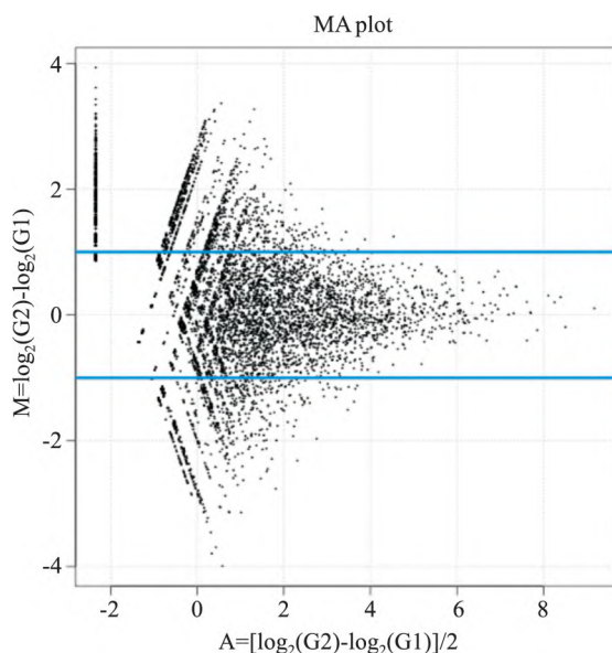
图6 NC与T2DM的外周血 circRNAs 的差异表达的 MA plot
