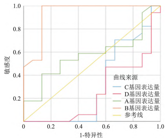
图7 所选定的4条 circRNA 的 ROC 曲线
