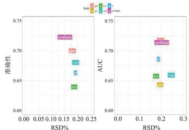
图 3 分类模型稳定性评估
