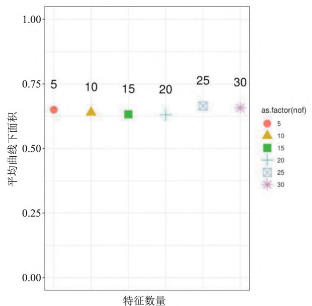
图 2 选择不同选定特征时所有分类器的平均 AUC
