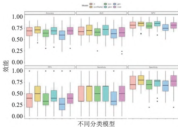
图4 分类模型交叉验证结果
